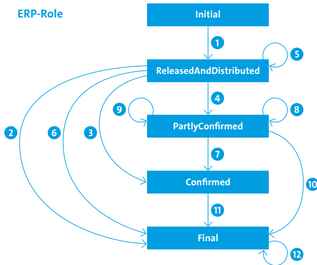
Abbildung 7: Zustandsdiagramm für den Hauptzustand der ERP-Rolle in der ERP-MES-Interaktion.
