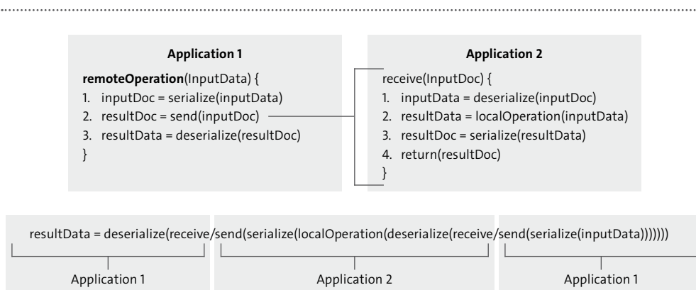
Abbildung 4: Ein entfernter Operationsaufruf verpackt die Serialisierung/Deserialisierung der transportierten Daten sowie den Datentransport und seine lokale Verarbeitung in einer Reihe von hintereinander ausgeführten Operationen. Diese werden einmal unter Verwendung von lokalen Variablen (oben) und ohne lokale Variablen (unten) dargestellt.
